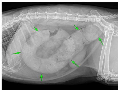
Afbeelding 2 Dilatatie colon
